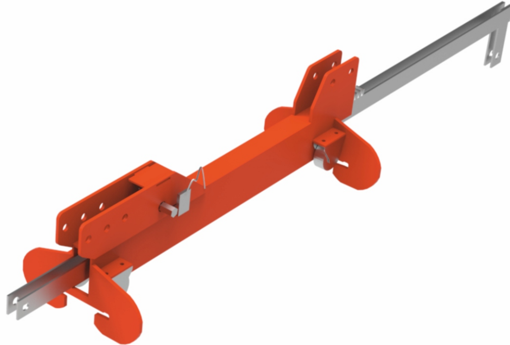
OCF Kalıp Kaydırma Mekanizması OCF Formwork Carrier
