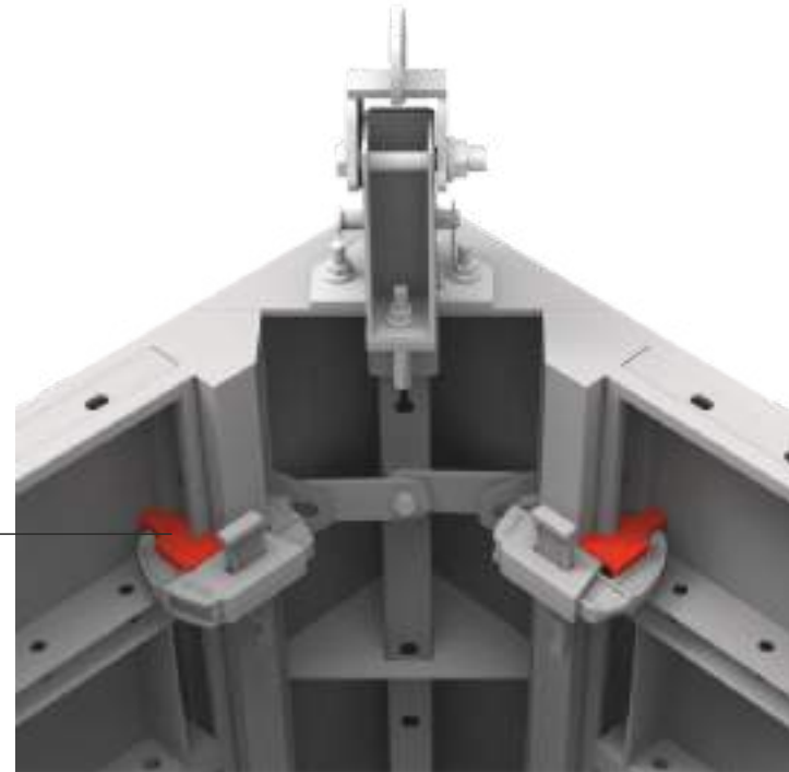
Rapid - Rapido Bağlantı Elemanı Rapid - Rapido Connector
